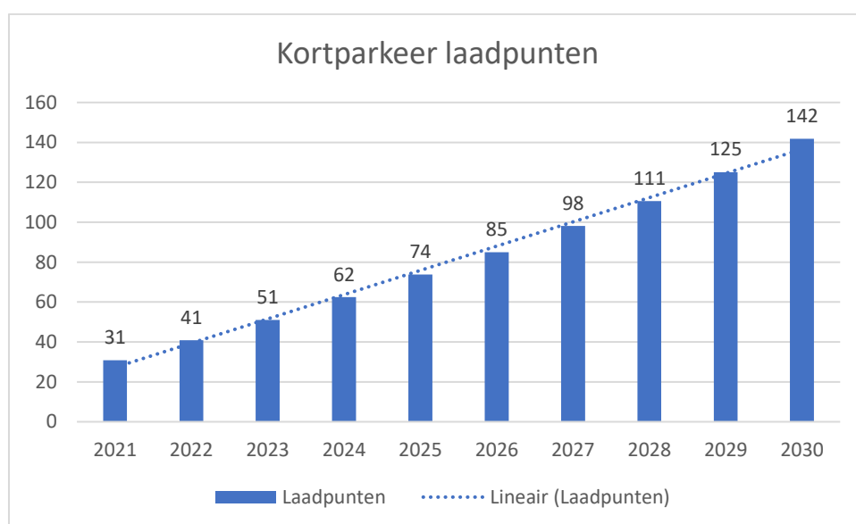
Figuur 5 Prognose kortparkeerlaadpunten (NAL-West)
